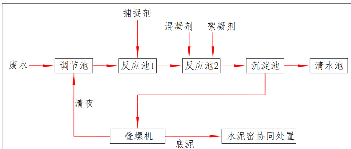
图 3.4-51 废水处理工艺流程
