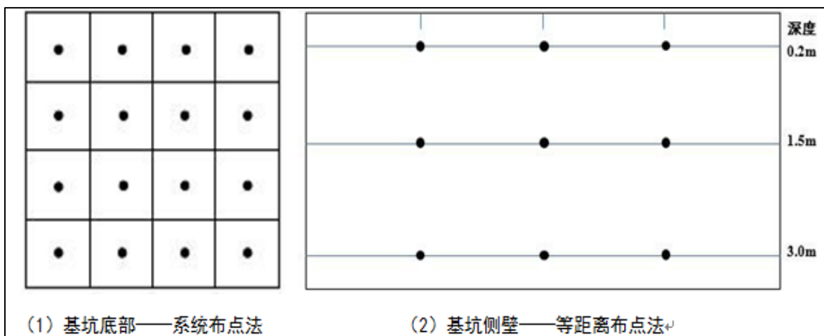
图 5.1-1 基坑底部与侧壁布点示意
