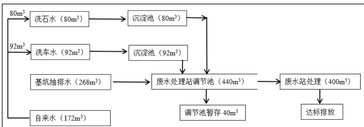
图 3.4-52 第一阶段项目水平衡图
